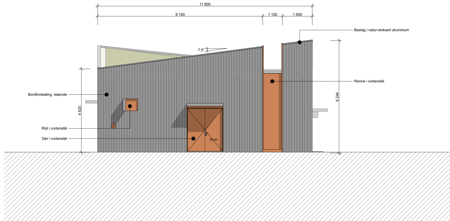
Fasade Sør
