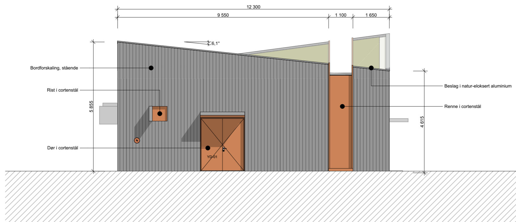
Fasade Nordøst
