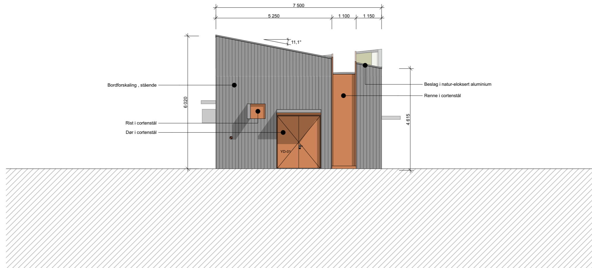
Fasade Sør
