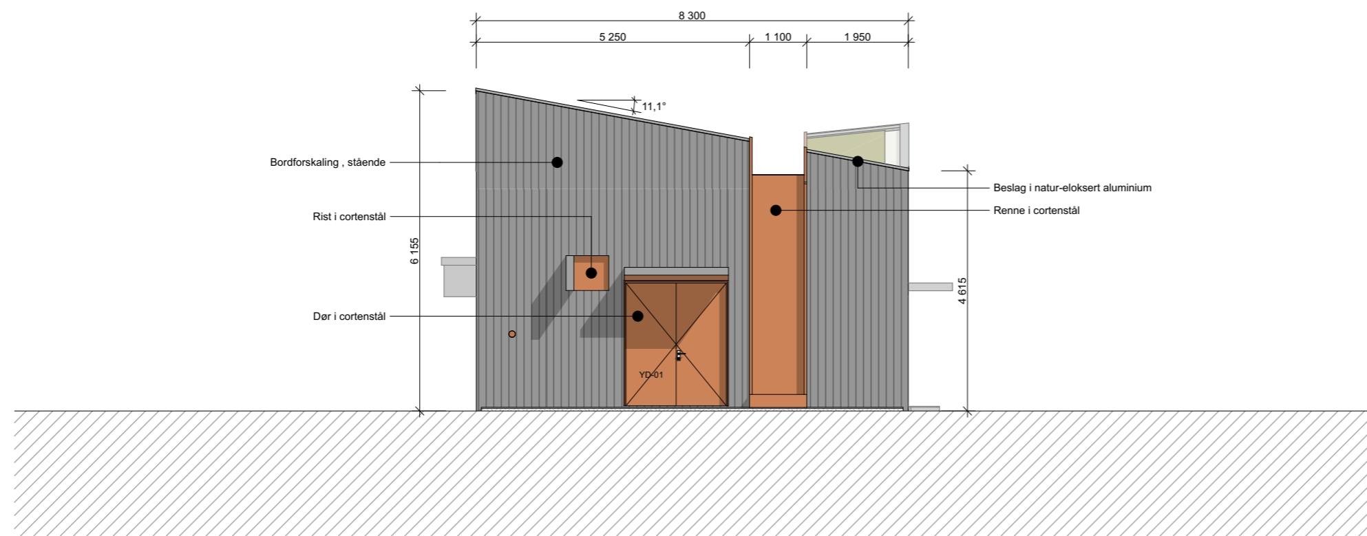
Fasade Sørøst
