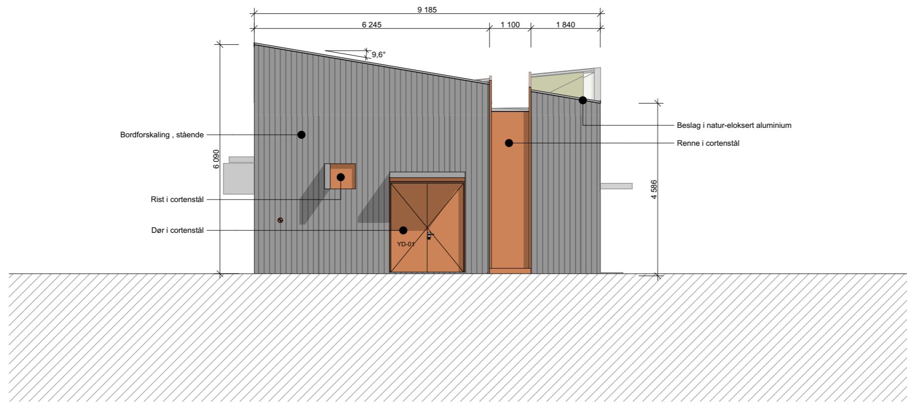
Fasade Sør
